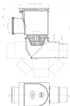
Schnitt A-A
